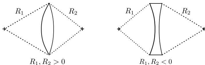
Obrázek 3: Konstrukce spojné a rozptylné čočky
