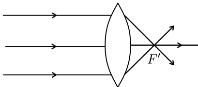
Obrázek 2: Lom svazku rovnoběžných paprsků na spojné čočce
