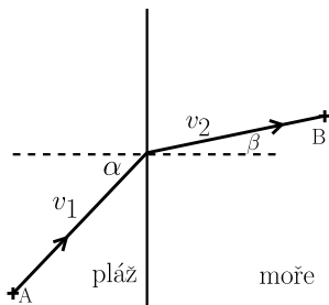
Obrázek 1: Znázornění nejrychlejší trajektorie z místa A k topícímu se člověku v místě B . Při jiné trajektorii si buď prodlužujeme uraženou dráhu, nebo strávíme příliš mnoho času plaváním.
