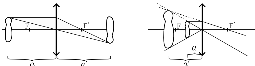
Obrázek 4: Zobrazení předmětu na spojně čočce ve dvou různých polohách vůči ohnisku
