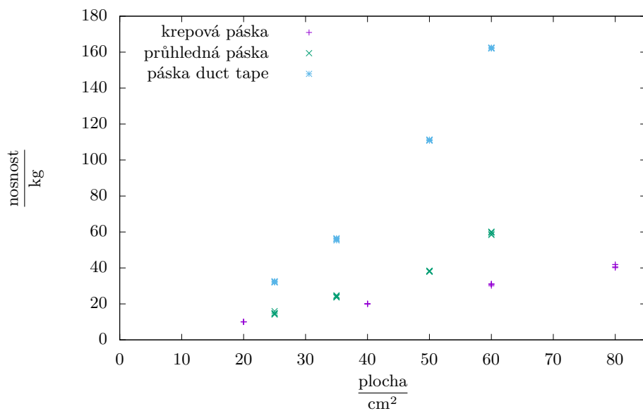
Obrázek 1: Graf závislosti nosnosti izolepy na použité ploše
