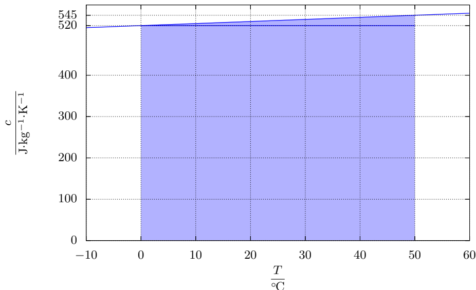
Obrázek 2: Graf měrné tepelné kapacity lineárně závislé na teplotě
