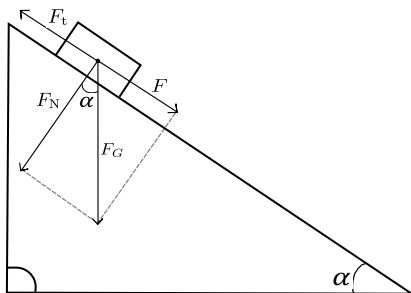
Obrázek 1: Znázornění sil působících na těleso na nakloněné rovině.
