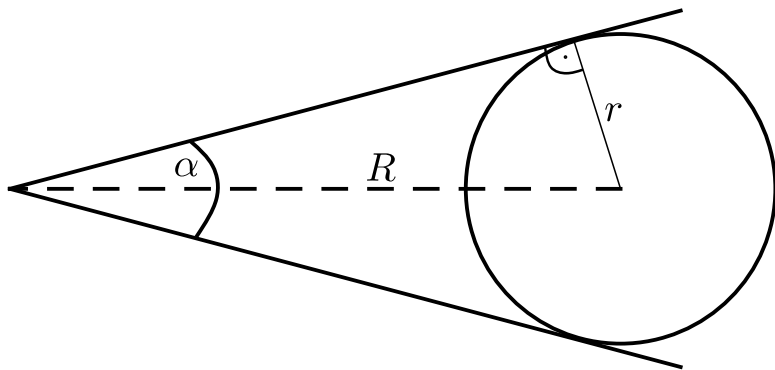
Obrázek 1: Pozorovaná úhlová velikost \alpha hvězdy s poloměrem r ze vzdálenosti R .
