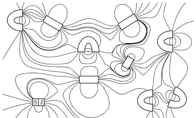
Obrázek 1: Magnety neznámé magnetizace
