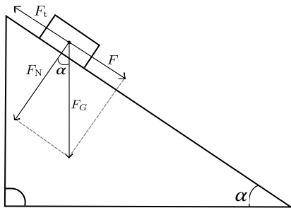
Obrázek 3: Znázornění sil působících na těleso na nakloněné rovině.
