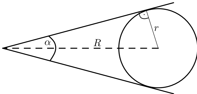
Obrázek 2: Pozorovaná úhlová velikost \alpha hvězdy s poloměrem r ze vzdálenosti R .
