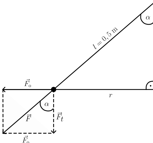
Obrázek 1: Kulička na provázku spolu s působícími silami
