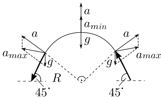
Obrázek 1: Trajektorie stíhačky.
