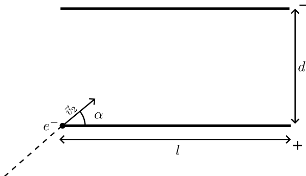
Obrázek 2: Elektrony letící pod úhlem \alpha
