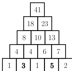
Obrázek 4: a = 1 a c = 2
