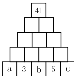
Obrázek 2: Pyramida s neznámými
