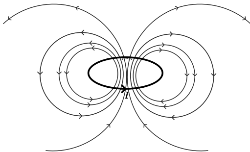
Obrázek 4: Magnetické siločáry v okolí proudové smyčky.
