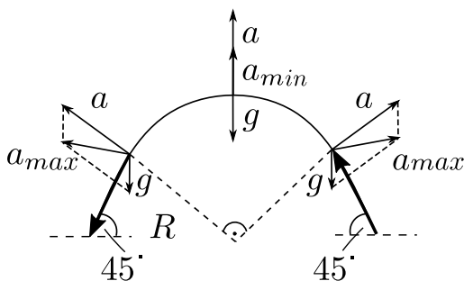
Obrázek 8: Trajektorie stíhačky.
