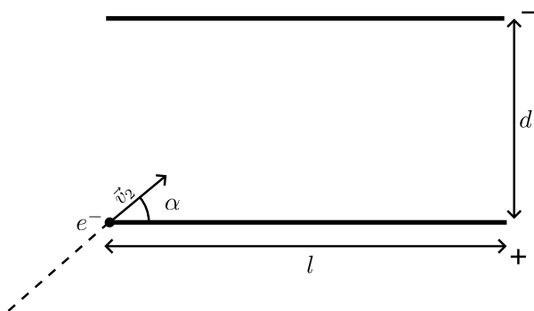
Obrázek 3: Elektrony letící pod úhlem \alpha
