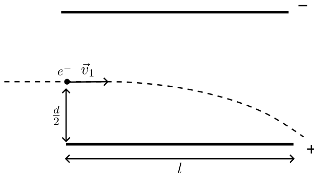
Obrázek 2: Elektrony letící rovnoběžně
