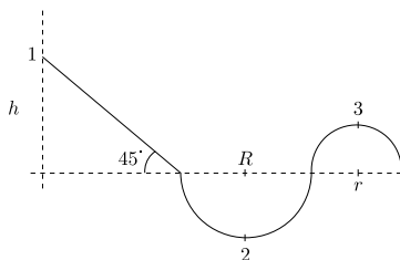
Obrázek 6: Vozík na horské dráze
