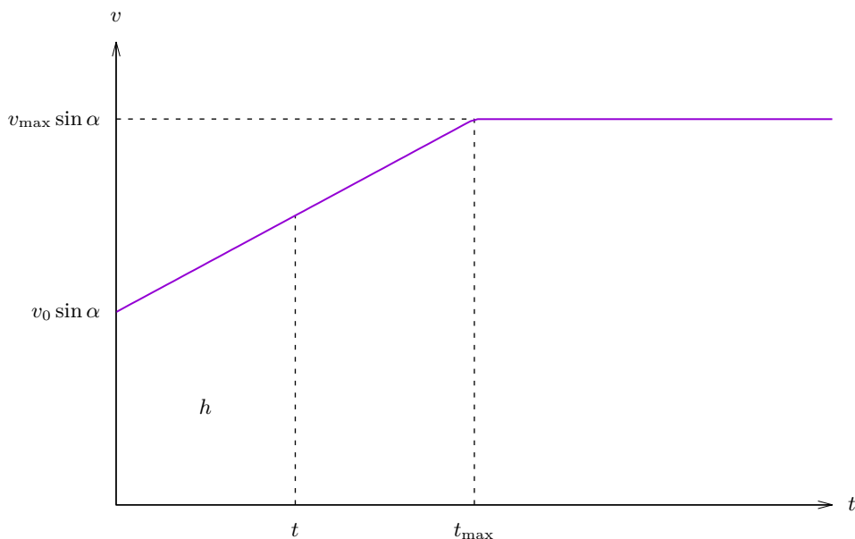
Obrázek 3: Graf znázorňuje závislost svislé složky rychlosti letadla na čase, plocha pod tímto grafem pak vyjadřuje změnu výšky. V této možnosti uvažujeme, že se letadlo dostane do výšky h ještě před dosažením maximální rychlosti.
