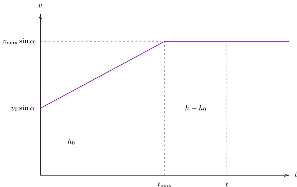
Obrázek 4: Graf znázorňuje případ, kdy letadlo dosáhne maximální rychlosti (v čase t_{\max} ) ještě před vystoupením do výšky h . Zbytek cesty proto urazí rovnoměrným pohybem.
