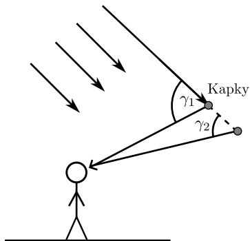
Obrázek 3: Schématické znázornění vzniku duhy. Sluneční paprsky dopadají na kapky pod nějakým úhlem daným výškou Slunce nad obzorem a po průchodu kapkou se odkloní o úhel \gamma . Když tedy pozorujeme duhu, díváme se na zlomené sluneční paprsky. Jak uvidíme v následující sekci, úhel \gamma závisí na vlnové délce (barvě) světla, proto na duze vidíme různé barvy v různých výškách nad obzorem.
