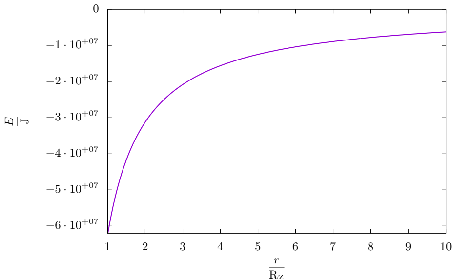
Obrázek 3: Graf potenciální energie gravitačního pole Země pro těleso o hmotnosti m = 1 kg.
