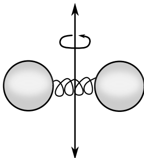
Obrázek 4: Klasická představa dvouatomové molekuly tvořené dvěma kuličkami spojenými pružinkou. Na obrázku je znázorněna i jedna z os, v jejímž směru se molekula může pohybovat a kolem které se může otáčet.
