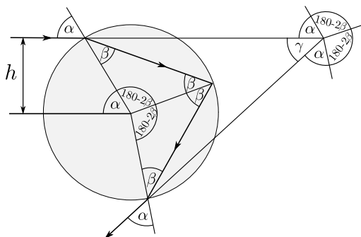
Obrázek 2: Lom paprsku kapkou vody
