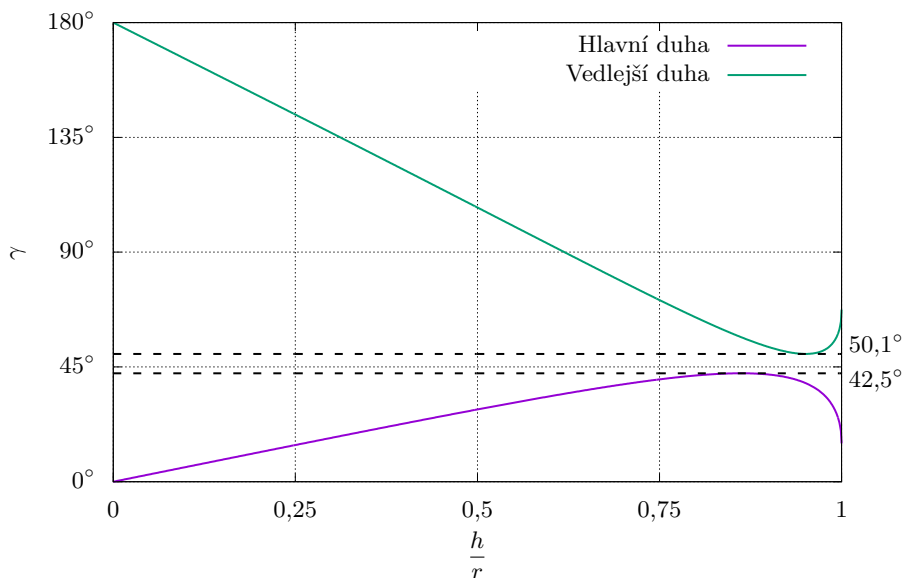
Obrázek 3: Závislost úhlu \gamma na poměru h/r pro primární a sekundární duhu
