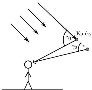
Obrázek 1: Schématické znázornění vzniku duhy. Sluneční paprsky dopadají na kapky pod nějakým úhlem daným výškou Slunce nad obzorem a po průchodu kapkou se odkloní o úhel \gamma . Když tedy pozorujeme duhu, díváme se na zlomené sluneční paprsky. Jak uvidíme v následující sekci, úhel \gamma závisí na vlnové délce (barvě) světla, proto na duze vidíme různé barvy v různých výškách nad obzorem.
