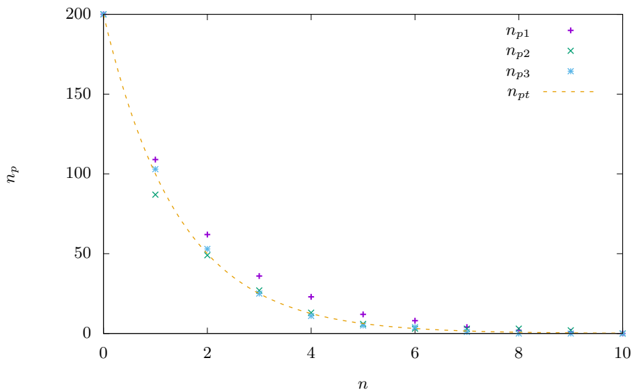
Obrázek 1: Počet čocky po n hodech s teoretickou závislostí n_{pt} . Teoretická závislost je pro přehlednost vyvedena spojitě.
