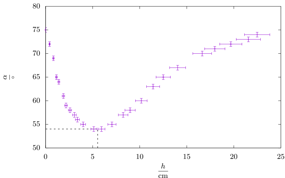
Obrázek 2: Závislost úhlu náklonu na výšce hladiny
