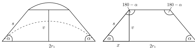
Obrázek 16: Řez komolým kuželem a náčrt lichoběžníka
