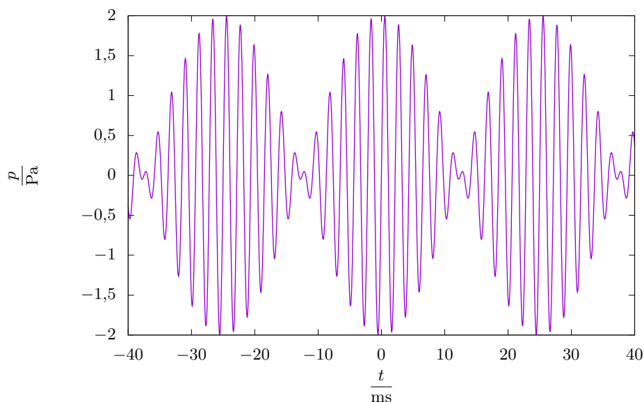
Obrázek 10: Záznej dvou tónů lišících se o 40 Hz
