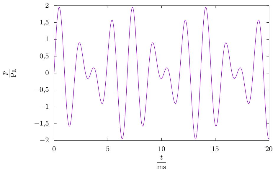
Obrázek 6: Graf závislosti akustického tlaku při souzvuku dvou tónů na čase
