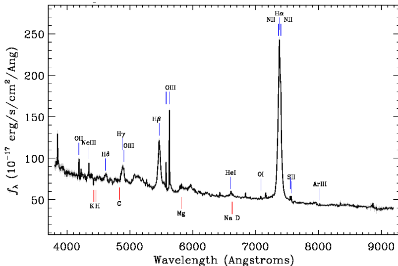
Obrázek 19: Závislost hustoty zářivého toku na vlnové délce s vyznačenými spektrálními čarami.
