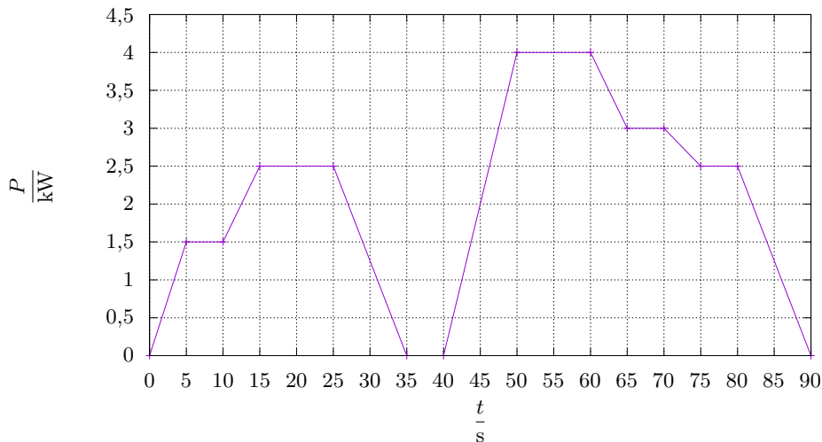
Obrázek 2: Průběh odebíraného výkonu navigáku v čase
