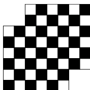
Obrázek 2: Upravená šachovnice
