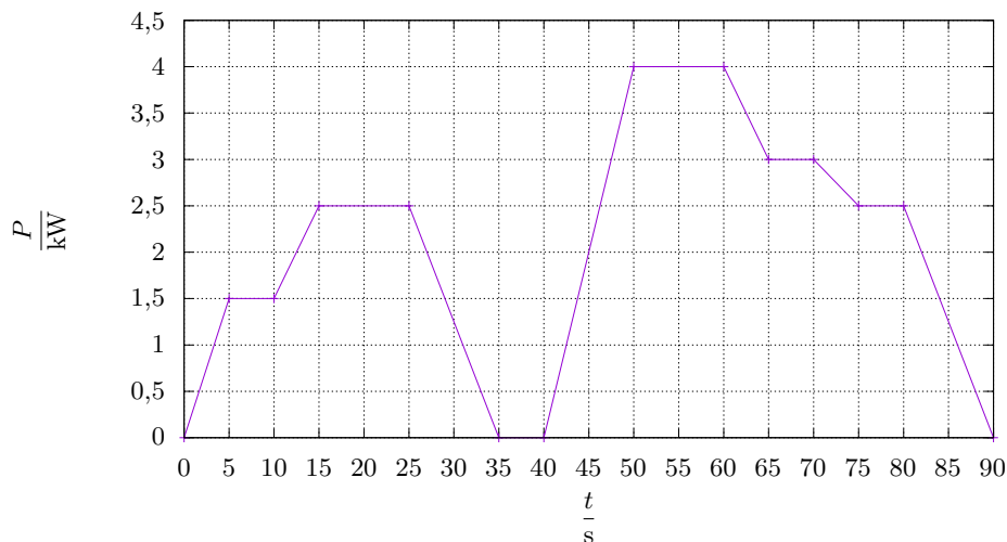
Obrázek 3: Průběh odebíraného výkonu navijáku v čase
