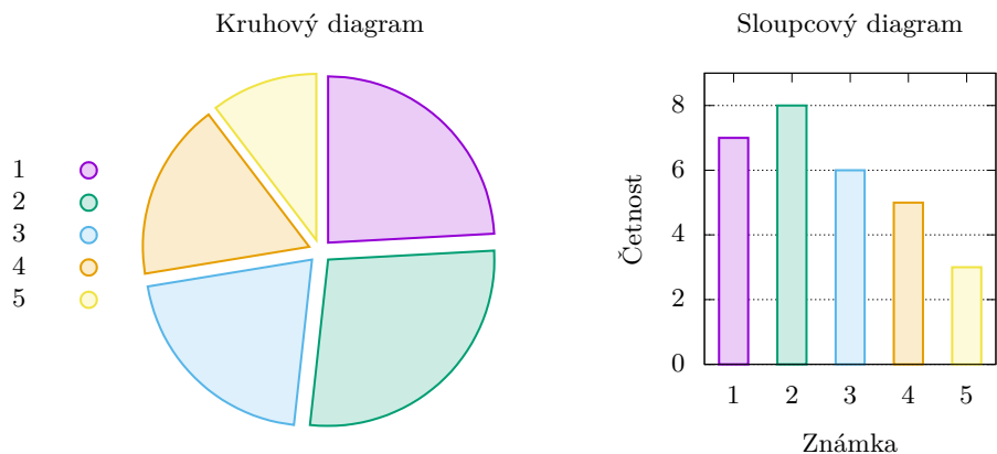
Obrázek 4: Porovnání zobrazení dat ve dvou typech diagramů na příkladu známek třídy z testu.
