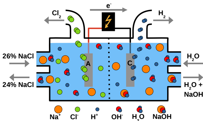
Obrázek 3: Schéma elektrolýzy vodného roztoku soli. Na anodě (na obrázku vlevo) se vylučuje plyný chlor, na katodě plyný vodík. Formuje se NaOH a je potřeba doplňovat jak roztok, tak vodu. Elektrody jsou oddělené stěnou, která propouští jen některé ionty. 10
