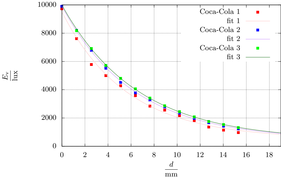
Obrázek 3: Závislost intenzity osvětlení na výšce Coca-Coly.
