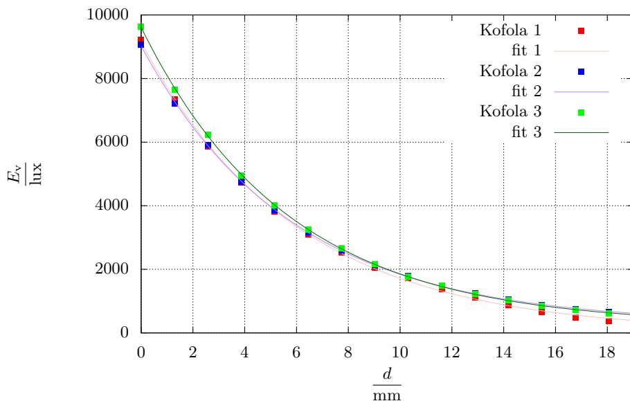
Obrázek 2: Závislost intenzity osvětlení na výšce Kofoly.
