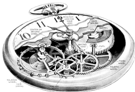
Obrázek 2: Diagram mechanických hodinek 4
